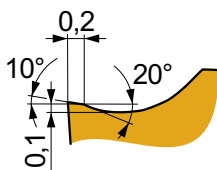
CNMG 120408E-FM
